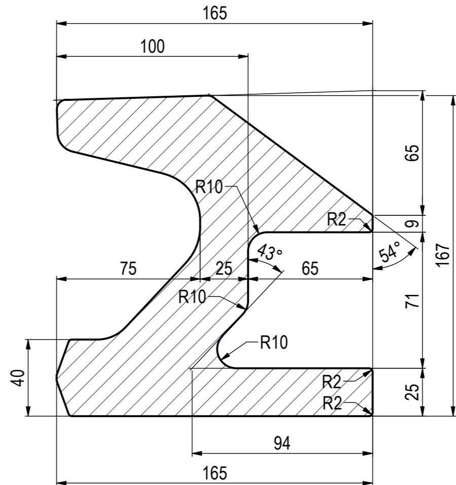
C-C (1:2)
