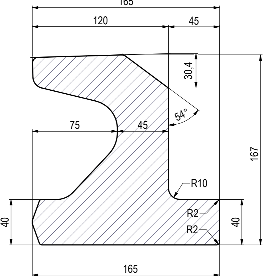
B-B (1:2)
