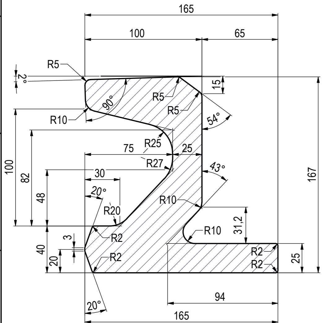
A-A (1:2)
