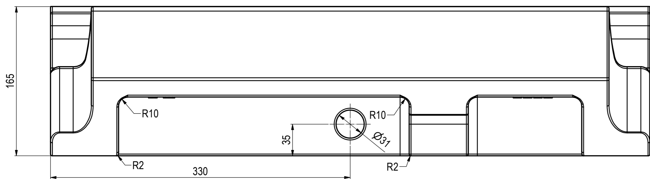
A-A (1:2)
