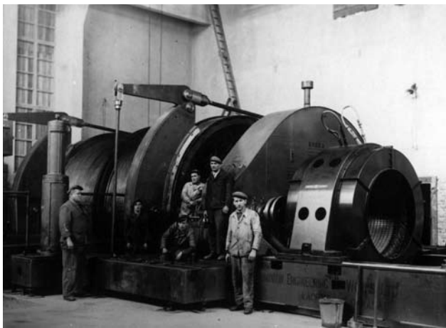
Monterji glavnega izvoznega stroja za prevažalni jašek v Starih Prelogah; stroj je danes na ogled na dvorišču Muzeja premogovništva Slovenije.
