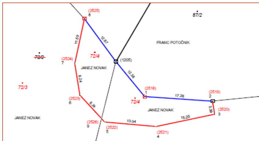
Primer ureditve meje in parcelacije
