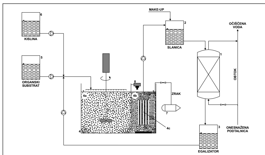
Shematski prikaz membranskega bioreaktorja za čiščenje podtalnice
