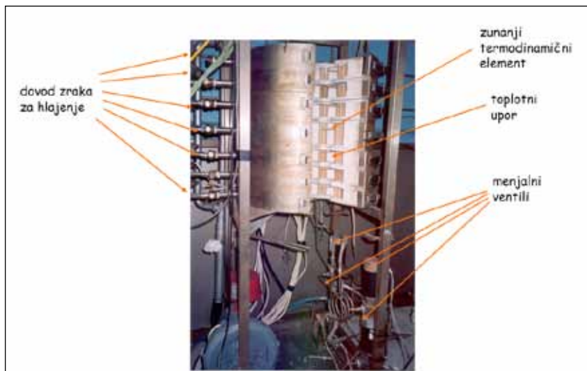
Preizkusna naprava Univerze v Oviedu za zajem metana
