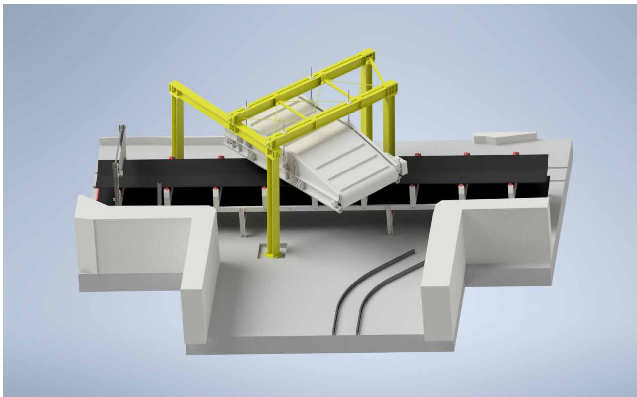
Situacija vgrajenega separatorja na transporterju T-60
