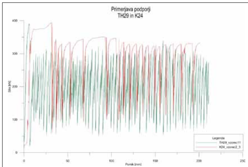
Primerjava popuščanja podporj K24 in TH29
