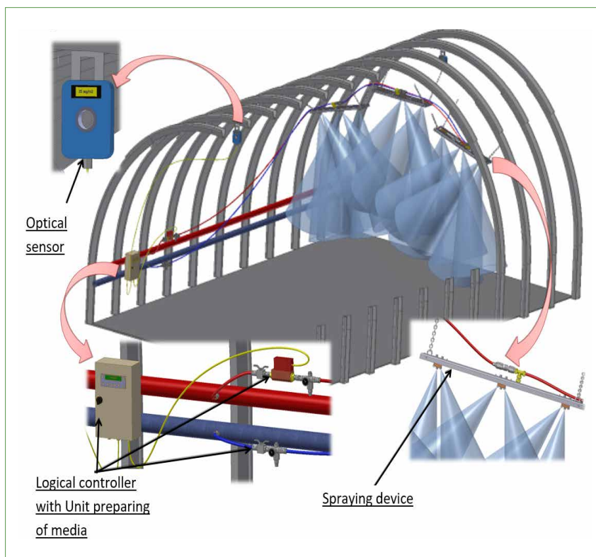
Pametna naprava s sistemom prh, krmiljena prek optičnega senzorja za meritve lebdečega prahu v jamskih progah, ki bo nadzoroval intenziteto delovanja prh, za optimalno pršenje glede na koncentracije prahu v zraku (KOMAG)
