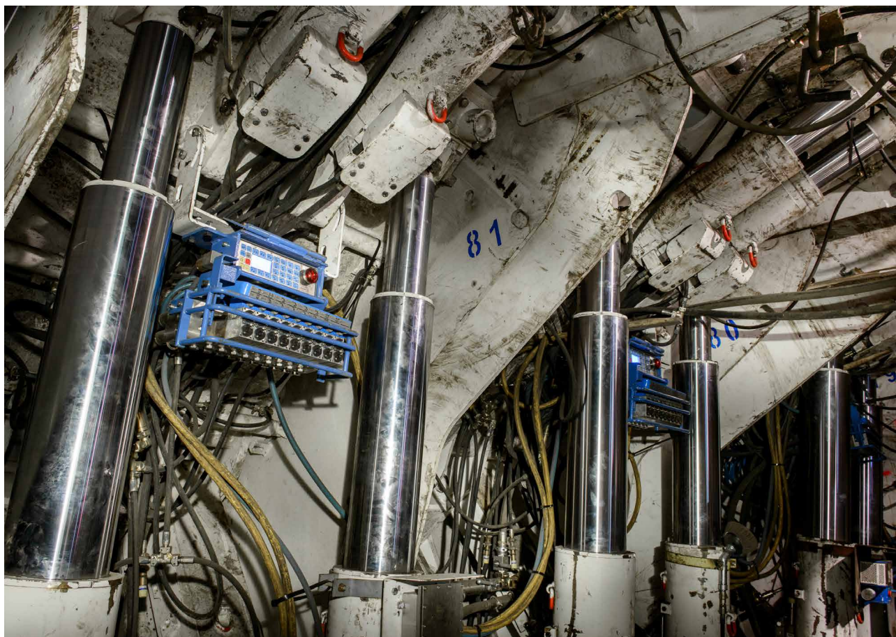
Na odkopu CD3G je vgrajena prva serija hidravličnega odkopnega podporja, razvitega in izdelanega v Premogovniku Velenje. (foto: Miran Beškovnik)
