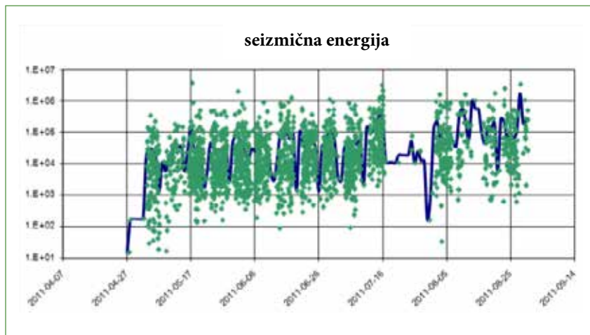
Grafični prikaz postopnega naraščanja seizmične energije med obratovanje odkopa C k. -50 v času izvajanja meritev
