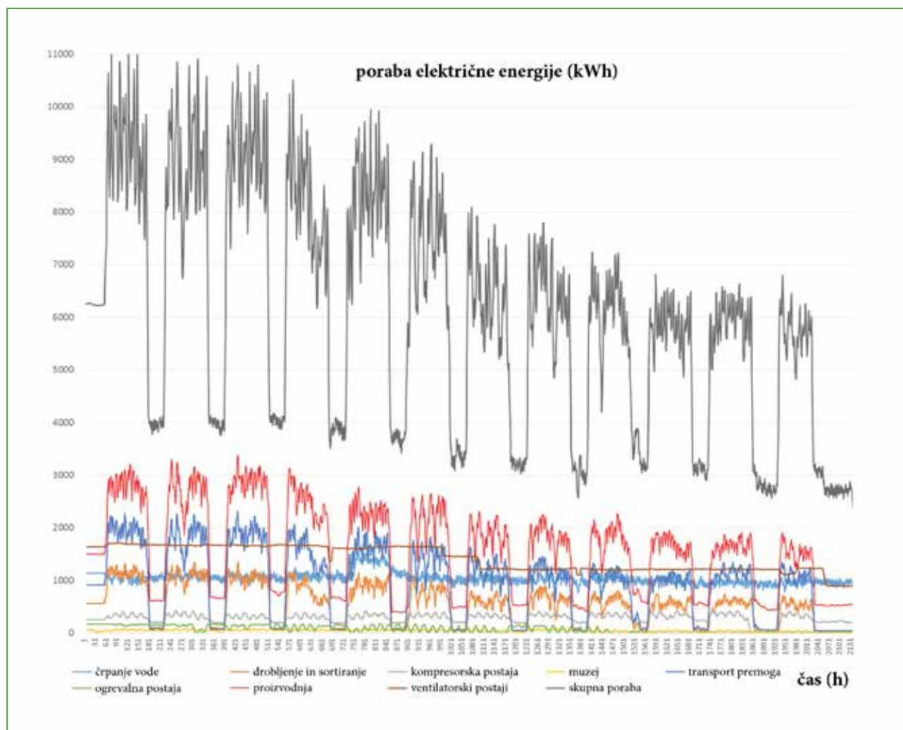
Grafični prikaz porabe električne energije v Premogovniku Velenje
