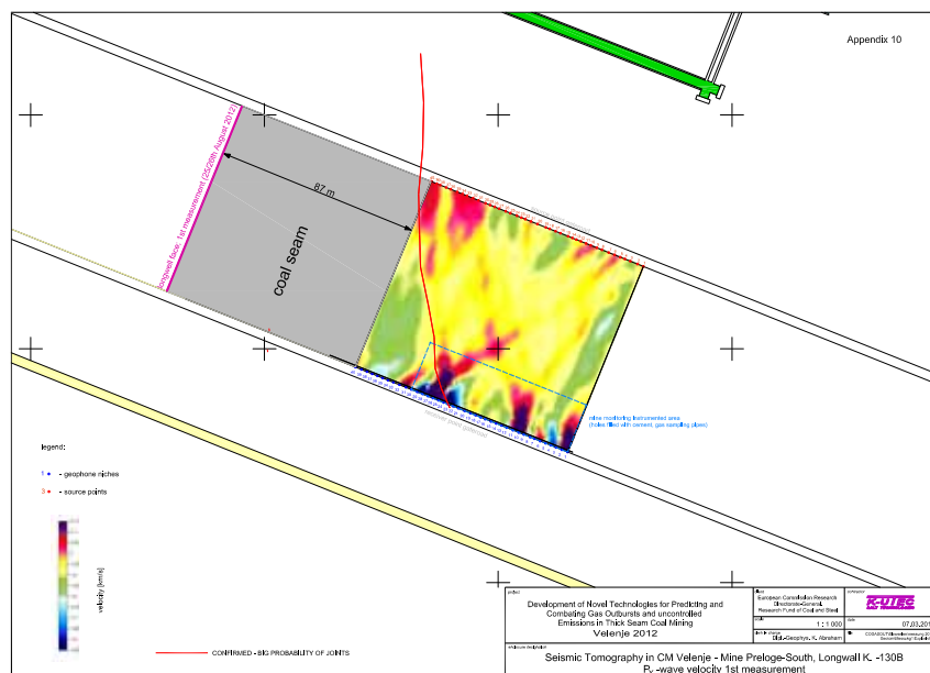
Interpretacija rezultatov izmerjenih hitrosti seizmičnih valov preko odkopnega stebra pri različnih oddaljenostih odkopa K. –130 B (Preiskave s seizmično tomografijo, K-UTEC)
