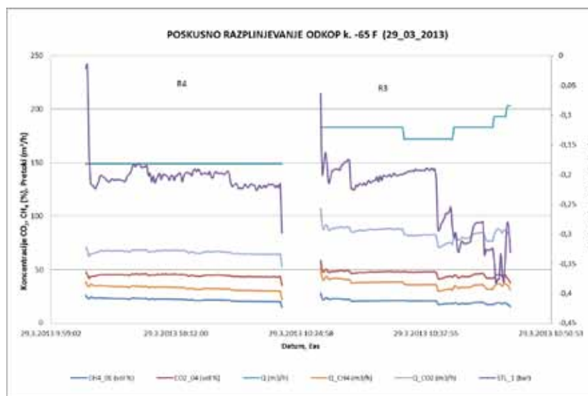
Diagram količin in koncentracij črpanega plina pri enem od poskusnih zagonov črpalke
