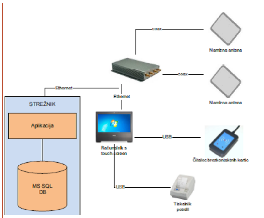
Shema sistema
