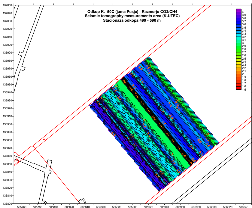
Prikaz razmerja koncentracij plinov v izstopnem zračilnem toku na odkopu K. -50 C v območju izvajanja seizmične tomografije
