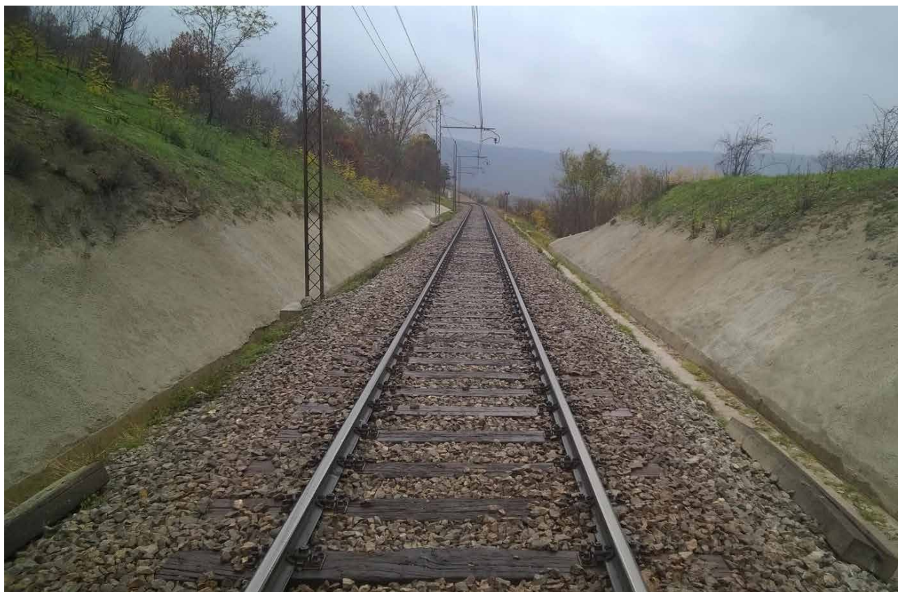
Končni videz protipožarnih presek po nanosu suhe betonske mešanice (SBS). (foto: Marko Ranzinger)
