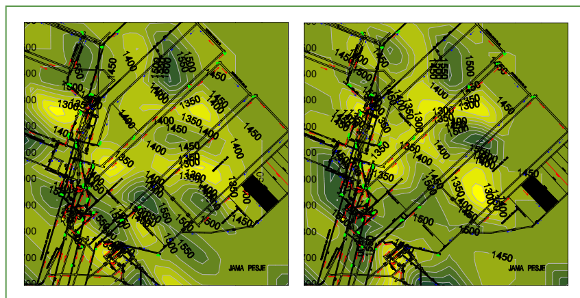
Slika 2: Primerjava hitrosti longitudinalnih valov (m/s) za prvo (levo) in drugo (desno) polovico septembra 2016; območja z večjimi hitrostmi predstavljajo lokacije koncentracije hribinskih napetosti.
