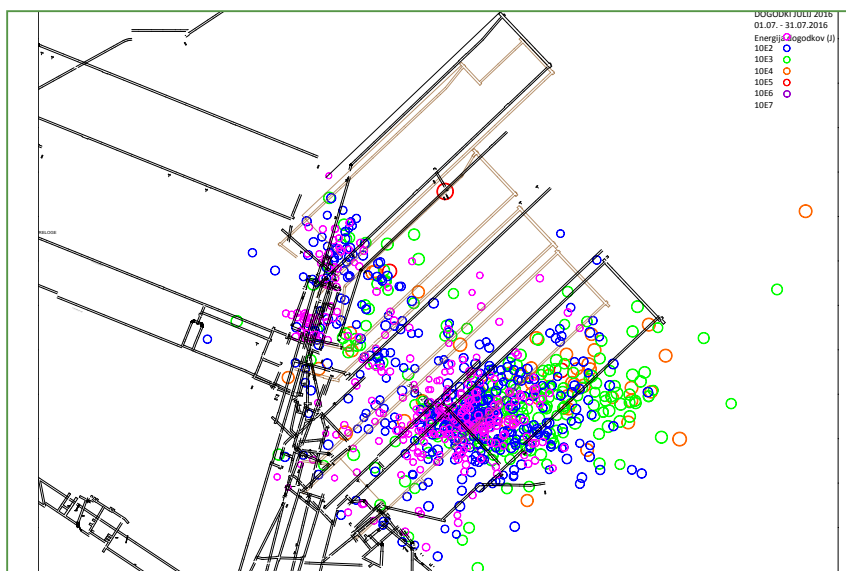
Slika 1: Zabeleženi seizmični dogodki v jami Premogovnika Velenje v juliju 2016
